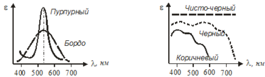
Рис.2. Виды полос поглощения окрашенных веществ
