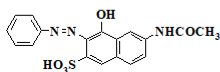
III б; Ярко-оранжевый краситель
