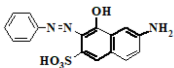
III а; Коричневато-оранжевый краситель
